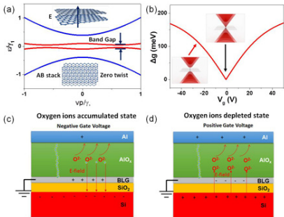
通过栅极电压调控存储窗口的原理图
